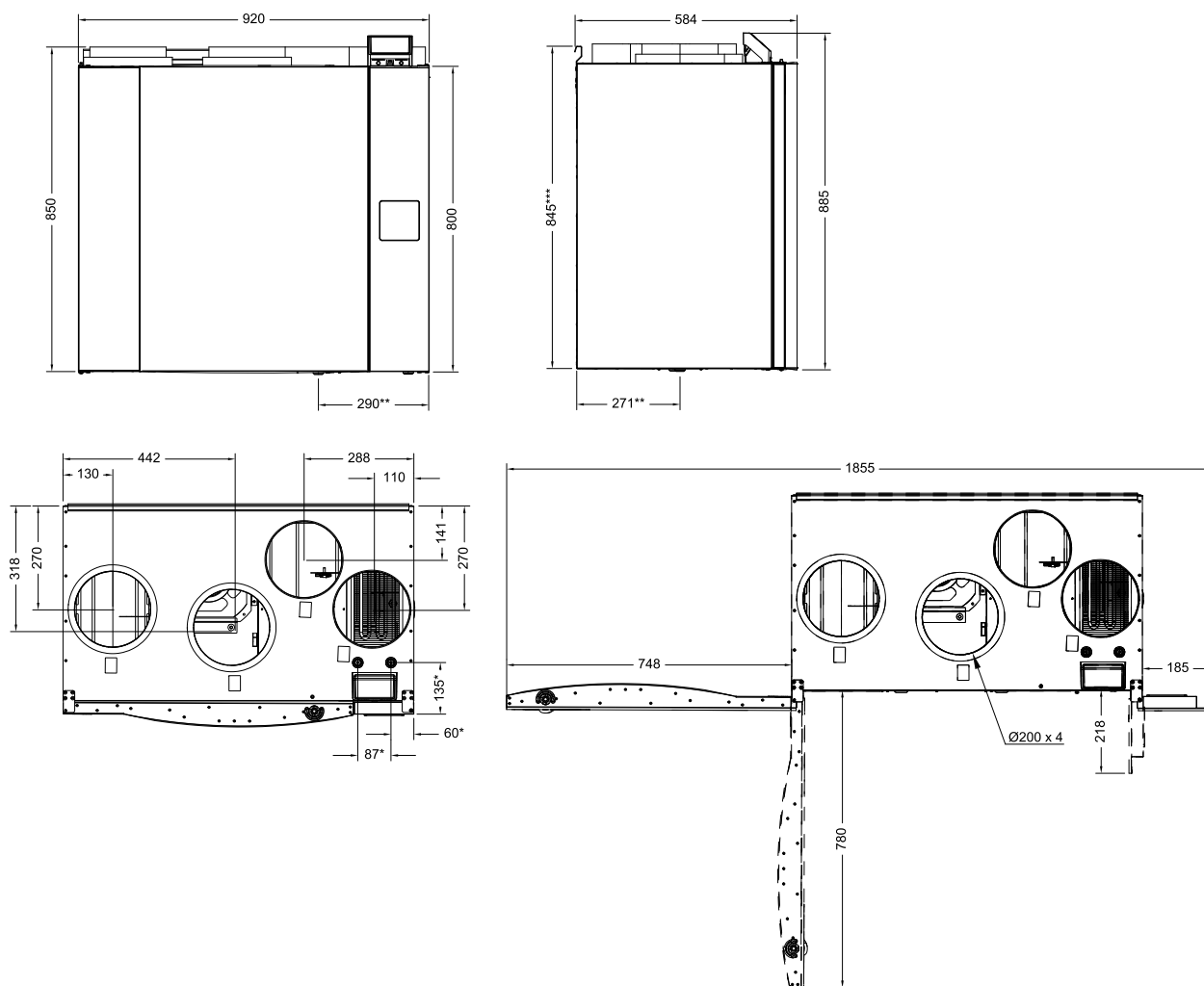
Fig. 3 Afmetingen en gewicht, R model
